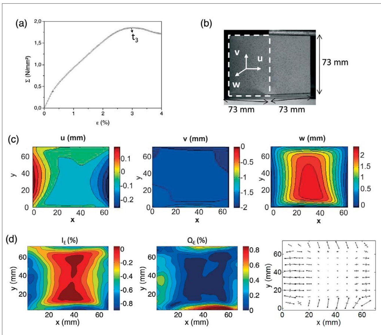
Figure 2 : (a) Courbe typique de compression d'une boîte : \Sigma = F/S_0 avec F la force de compression, S_0 la surface de la section du panneau, \epsilon = \Delta/h_0 avec h_0 la hauteur initiale de la boîte et h sa variation de hauteur. (b) Boîte en carton ondulé avec profil de cannelure G à la force de compression maximale enregistrée (point t_3 sur la courbe). Ses surfaces ont été recouvertes d'un mouchetis pour la stéréocorrélation d'images. (c) Composantes u , v et w du champ de déplacement d'un panneau (exprimé dans un repère local attaché à ce dernier). (d) I_E : déformation moyenne en traction/compression ou encore demi-variation surfacique relative, Q_E : déformation moyenne en cisaillement et représentation schématique de la direction et de l'intensité des déformations principales. Données correspondant à la force de compression maximale relevée au cours de la compression d'une boîte de 73 mm × 73 mm × 73 mm.
