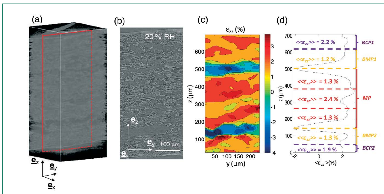
Figure 1 : (a) Visualisation 3D du carton plat à une humidité relative de 20%. (b) Coupe ( e_y, e_z ) selon l'épaisseur. (c) Carte de la composante \epsilon_{zz} du champ de déformation du carton plat évaluée à partir des déplacements mesurés dans le plan ( e_y, e_z ) pour une variation d'humidité relative de 20% à 50%. (d) Profil de déformation moyen \langle \epsilon_{zz} \rangle selon l'épaisseur et valeurs moyennes par couche.
